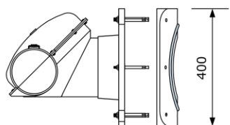
Type P1 med monteringsplate
